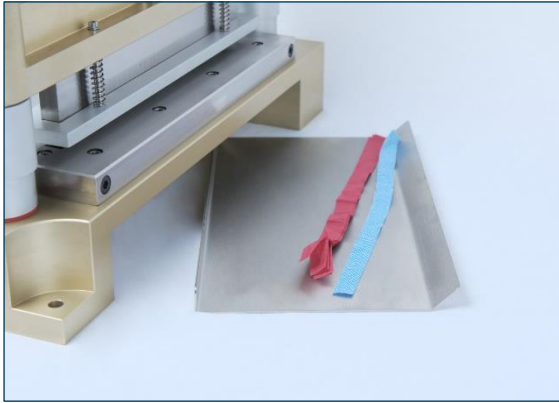
Probenauffangschale für einfache Entnahme
